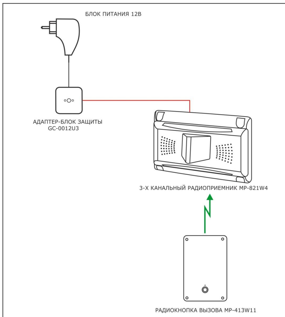
Рисунок 3.1. Структурная схема комплекта радиовызова MP-920W11
