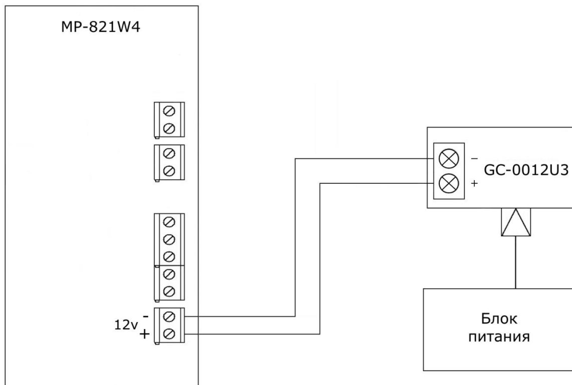
Рисунок 7.4. Схема соединений комплекта радиовызова MP-920W11
