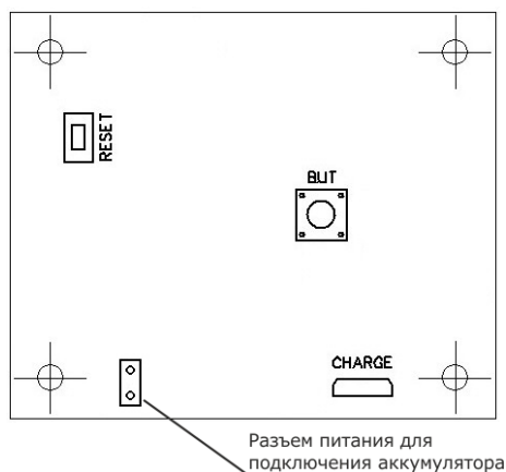
Рисунок 7.1. Внешний вид платы радиокнопки вызова MP-413W11
