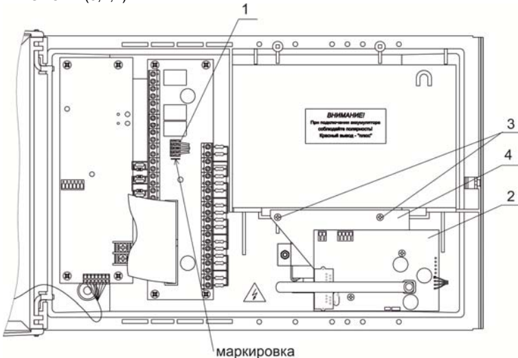
б) Установочное место модуля автодозвона ВЗРС-МАД в корпус приборов ВЗРС-ПК(16,24)
