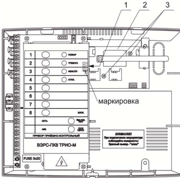
а) Установочное место модуля автодозвона ВЗРС-МАД в корпус приборов ВЗРС-ПК(8,4,2).
