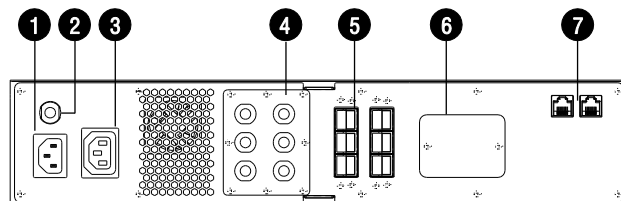
BP48VP2U04
