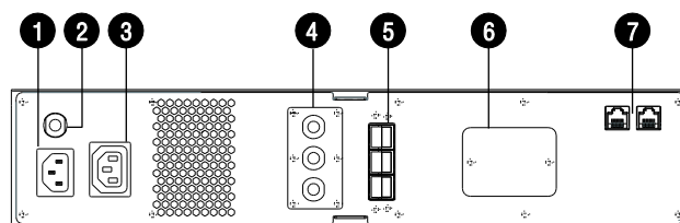
BP48VP2U03
