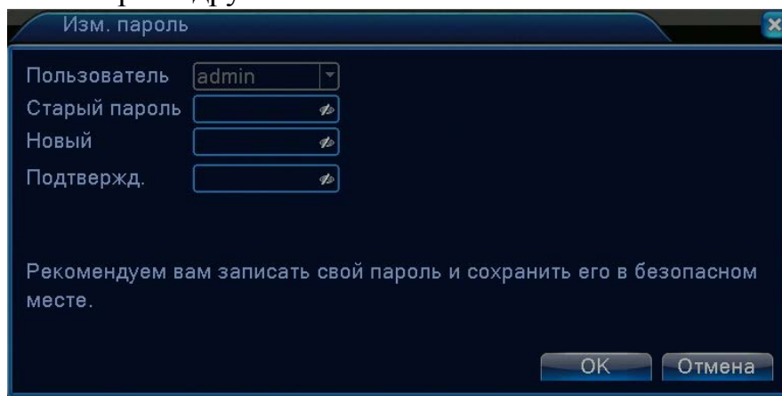
Рисунок 4.46 Изменить пароль
