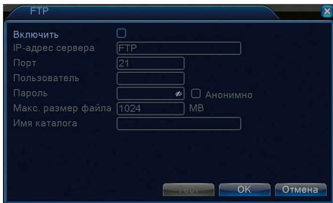
Рисунок 4.22 Настройки FTP
