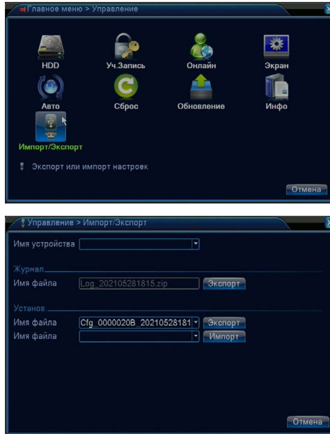
Рисунок 4.56 Интерфейс импорта/экспорта
