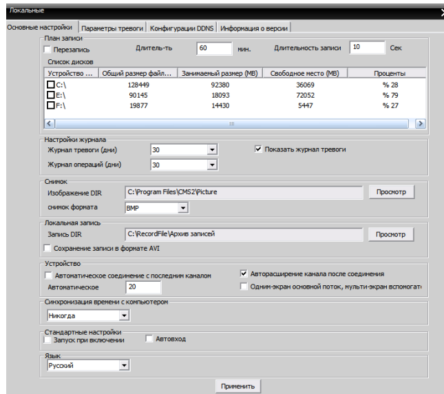
Рисунок 4.4 Настройки программы.
