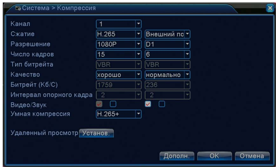
Рисунок 4.15 Настройки компрессии
