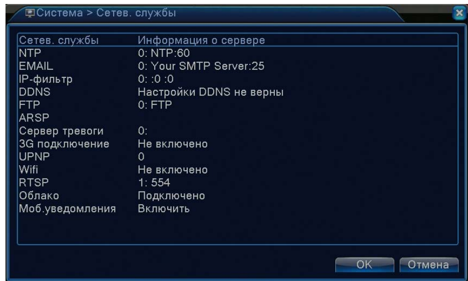
Рисунок 4.17 Сетевые службы
