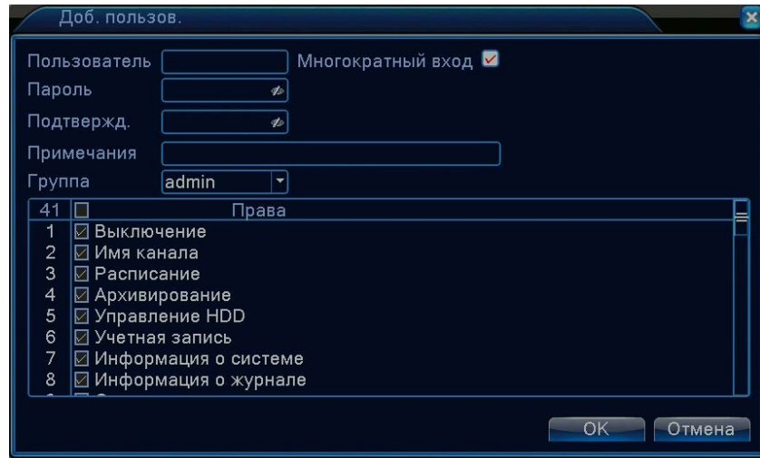
Рисунок 4.47 Добавить пользователя
