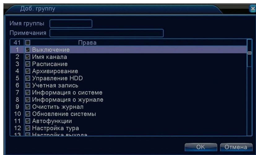
Рисунок 4.48 Добавить группу
