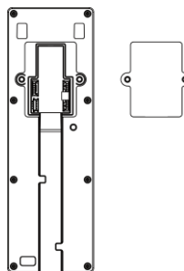
Рисунок 3-10. Снятие задней панели
