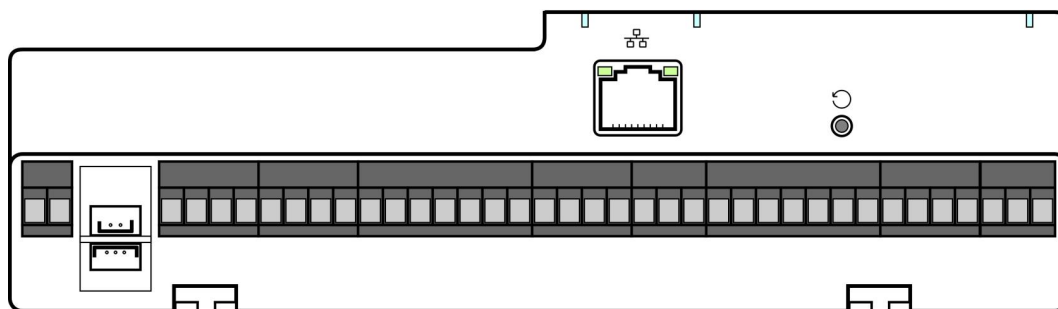
Схема расположения основных элементов на корпусе контроллера E4 Lite, вид сбоку.
