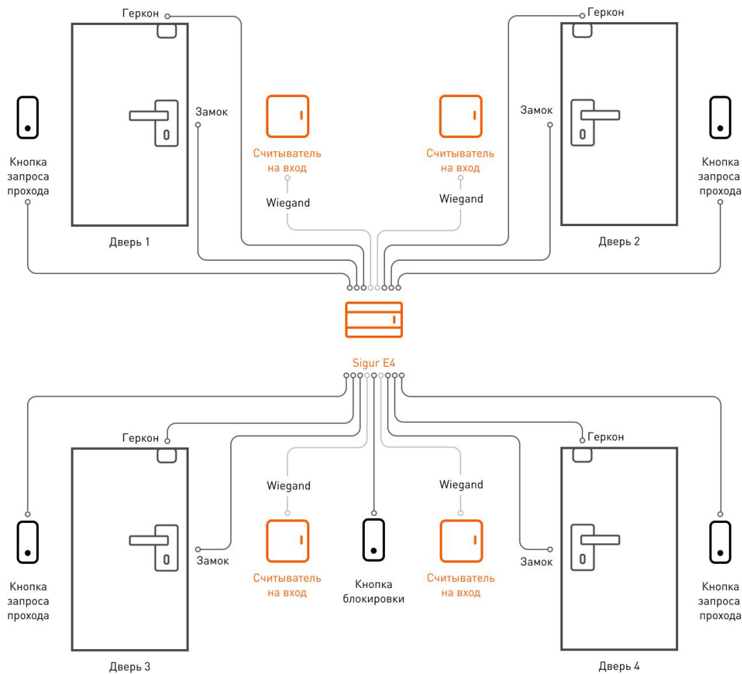
Пример подключения оборудования в конфигурации «Четыре двери, потенциальное управление».
