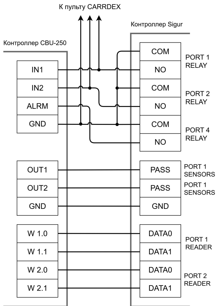
Электронные проходные CARDDEX, контроллер турникета CBU-250 (CBU-150/250).
