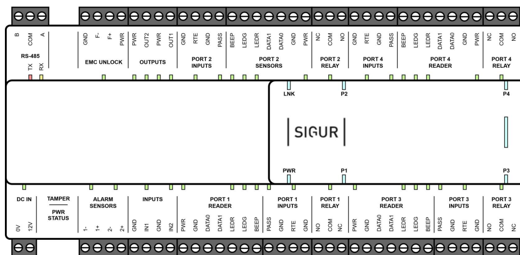
Схема расположения основных элементов на корпусе контроллера E4 Lite, вид сверху.
