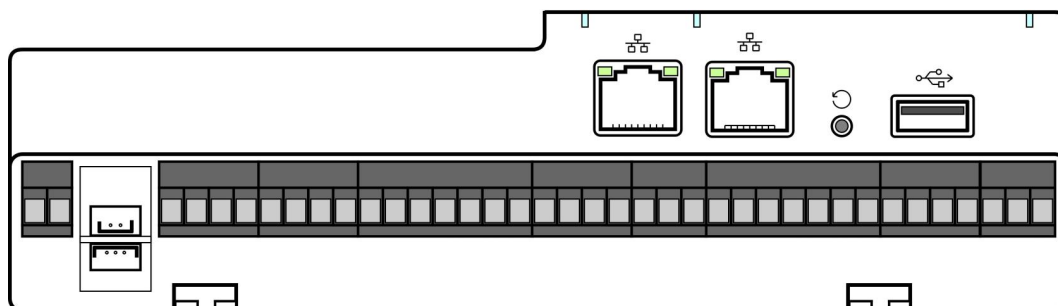
Схема расположения основных элементов на корпусе контроллера E4 Pro, вид сбоку.
