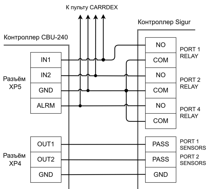
Подключение блока управления CBU-240.
