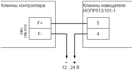
Подключение охранно-пожарного извещателя ИОПР513/101-1 к одному контроллеру.
