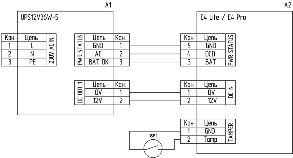
Схема электрическая принципиальная контроллера E4 Lite UPS и E4 Pro UPS.
