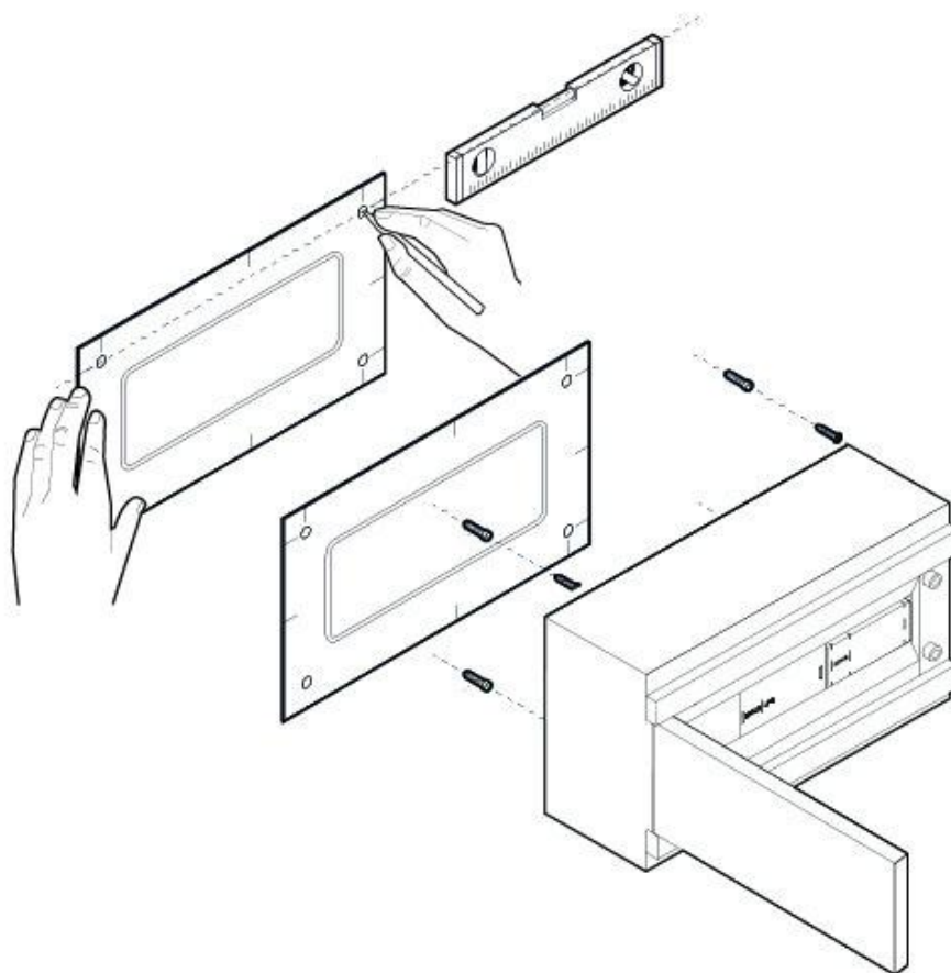
Монтаж контроллера.
