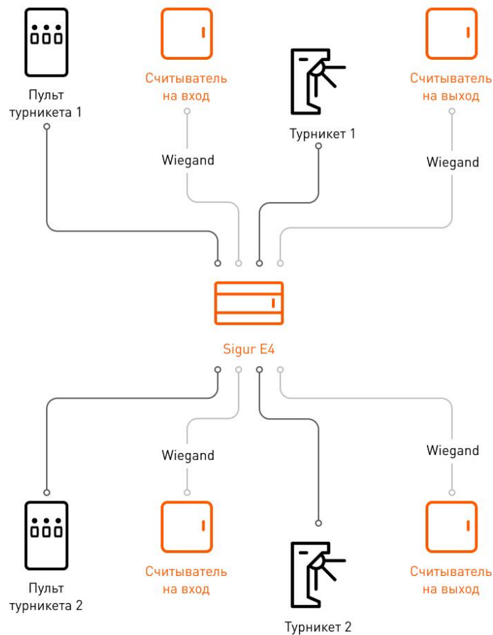
Вариант подключения в конфигурации «Два турникета, потенциальное управление».
