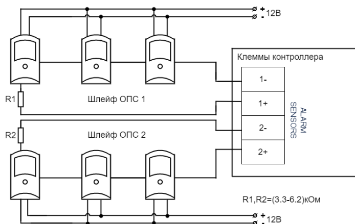
Подключение датчиков ОПС, требующих отдельного питания.
