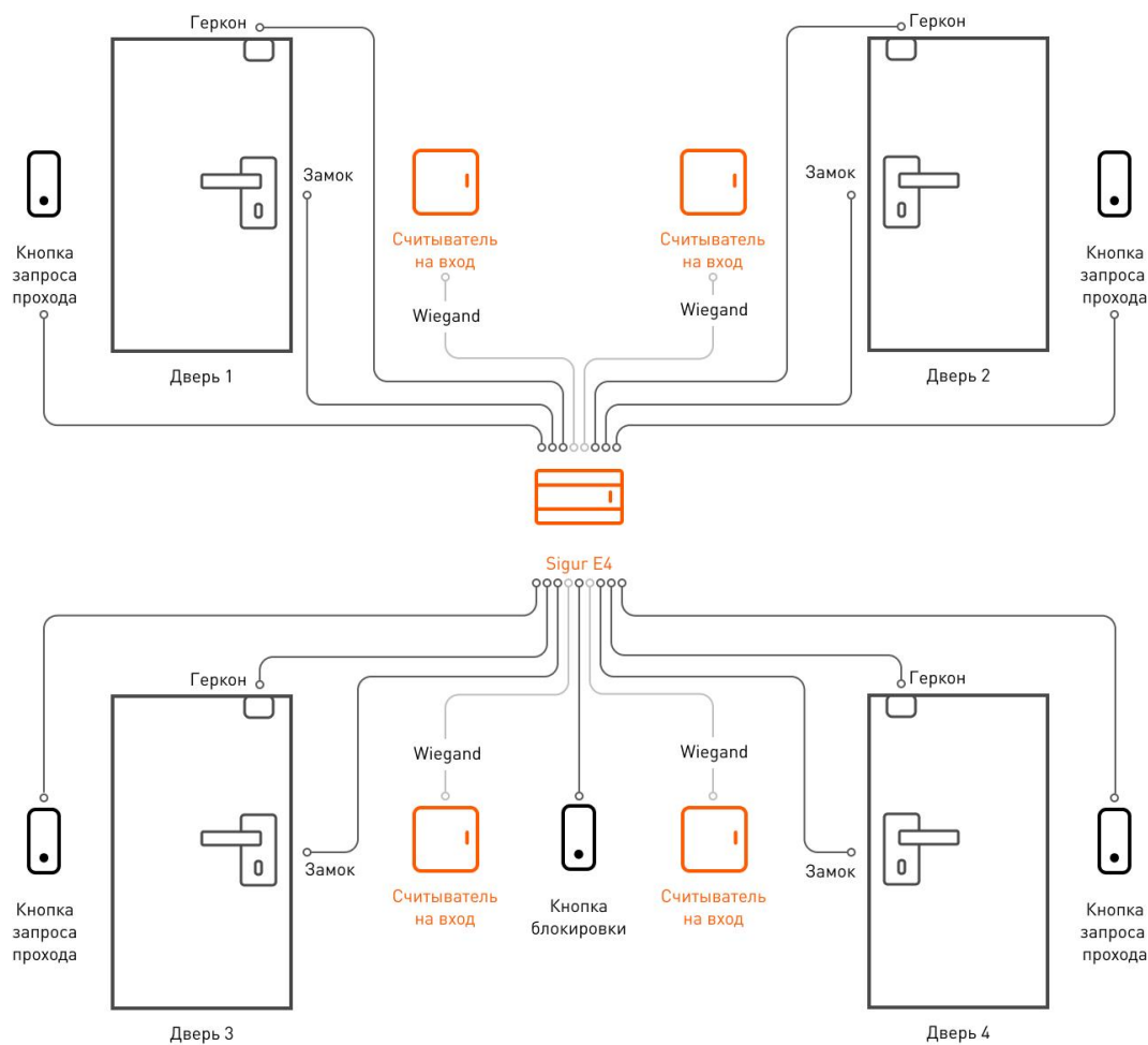
Пример подключения оборудования в конфигурации «Четыре двери, импульсное управление».
