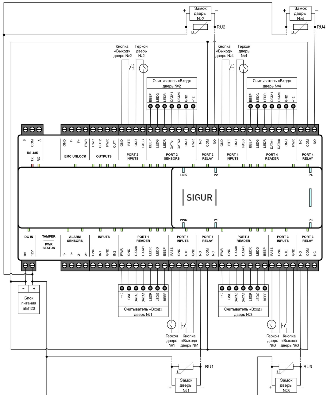
Пример подключения четырёх дверей.
