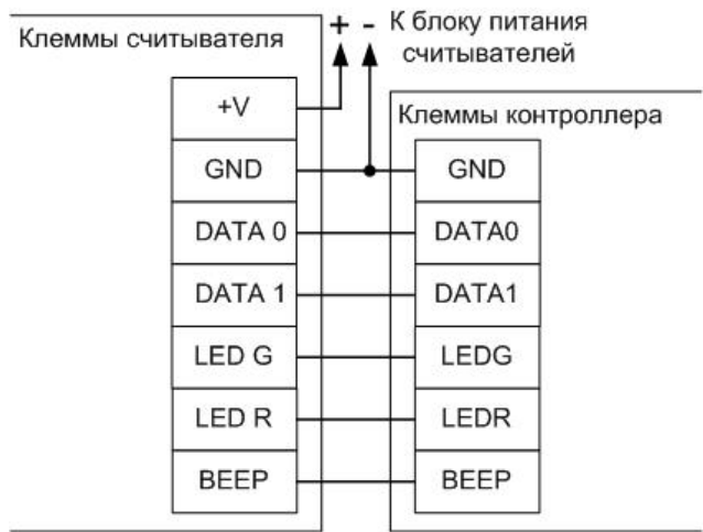
Пример подключения считывателя с напряжением питания, отличающимся от напряжения питания контроллера или считывателей, потребляющих ток больше 200 мА.
