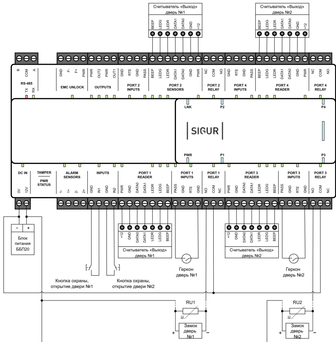
Пример подключения двух дверей.
