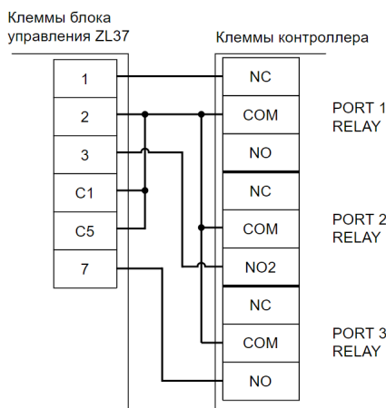
Схема подключения блока управления ZL37, ZL38.
