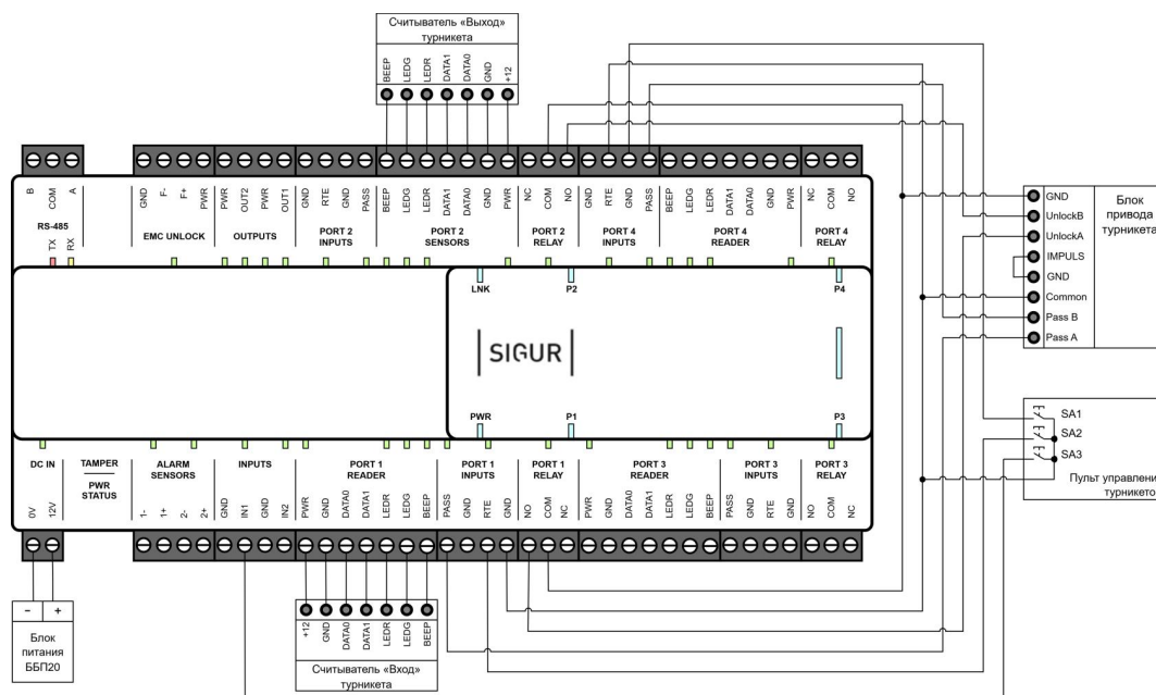
Пример подключения турникета.
