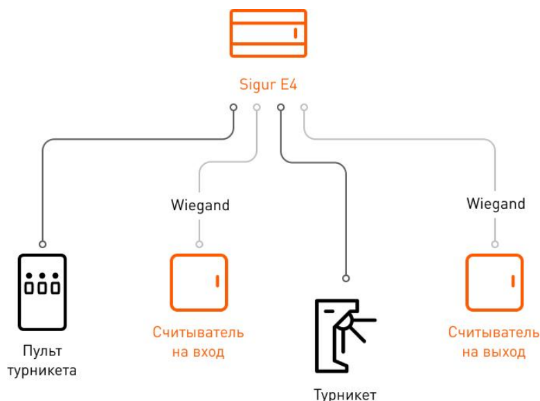
Вариант подключения в конфигурации «Турникет, потенциальное управление».
