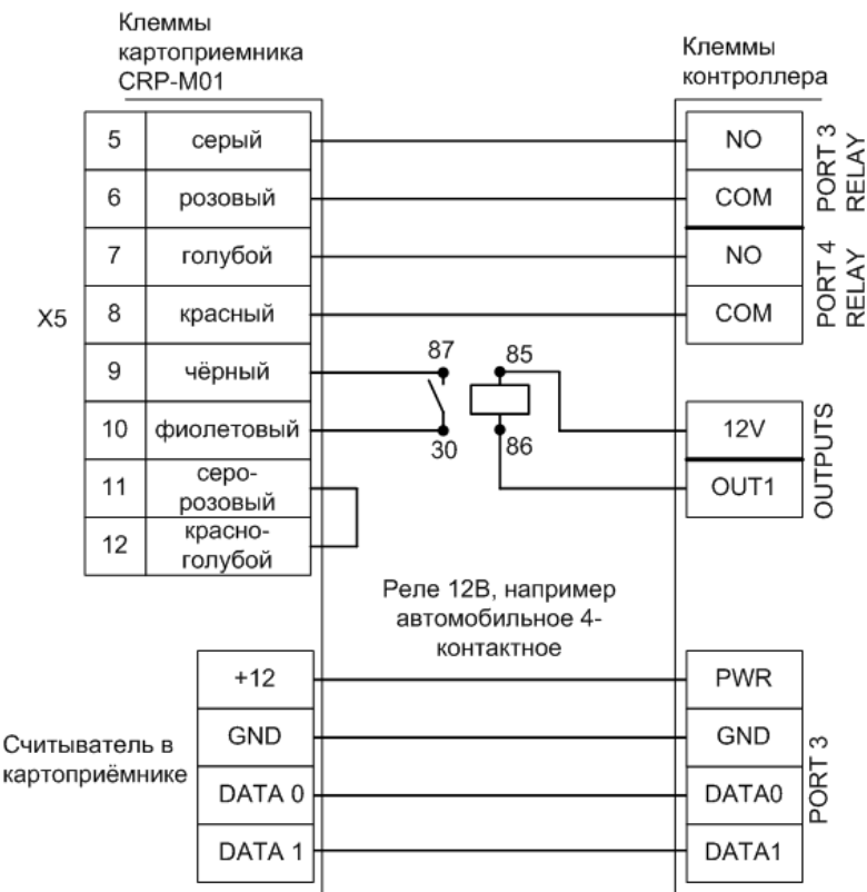
Пример подключения KABA CRP-M01.
