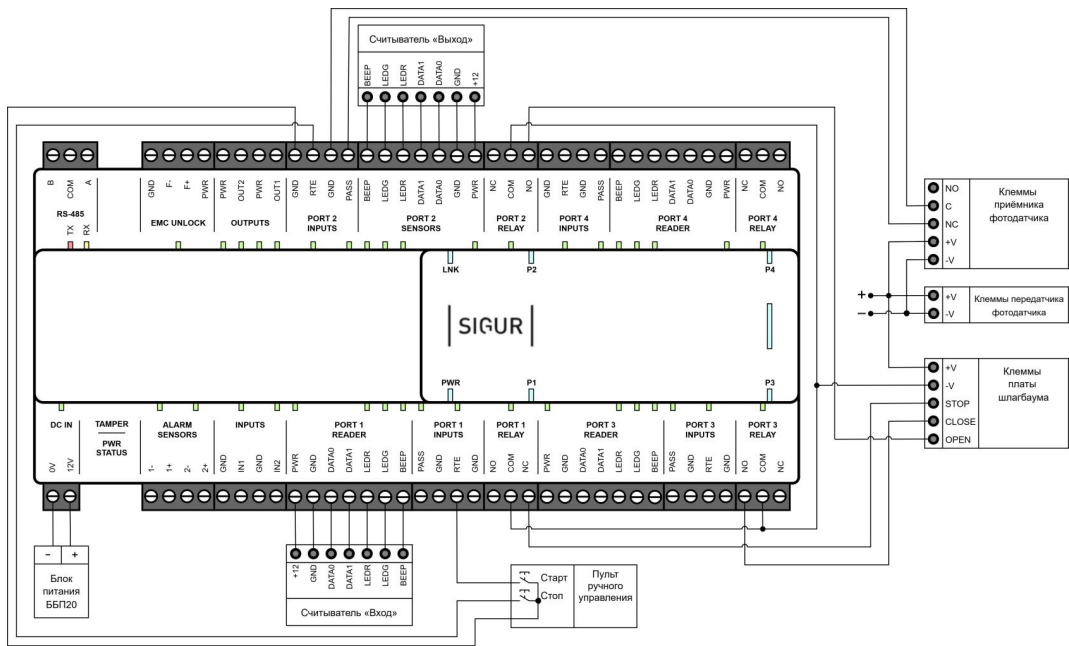
Пример подключения шлагбаума.
