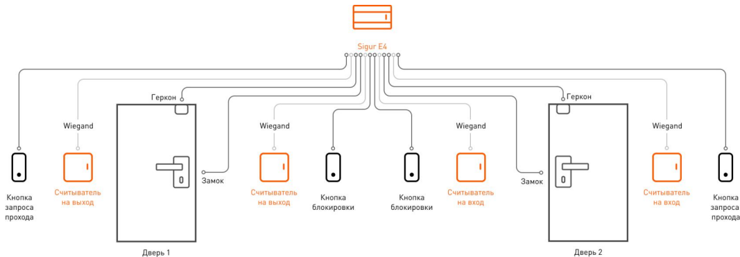
Вариант подключения комплекта оборудования в конфигурации «Две двери, импульсное управление».
