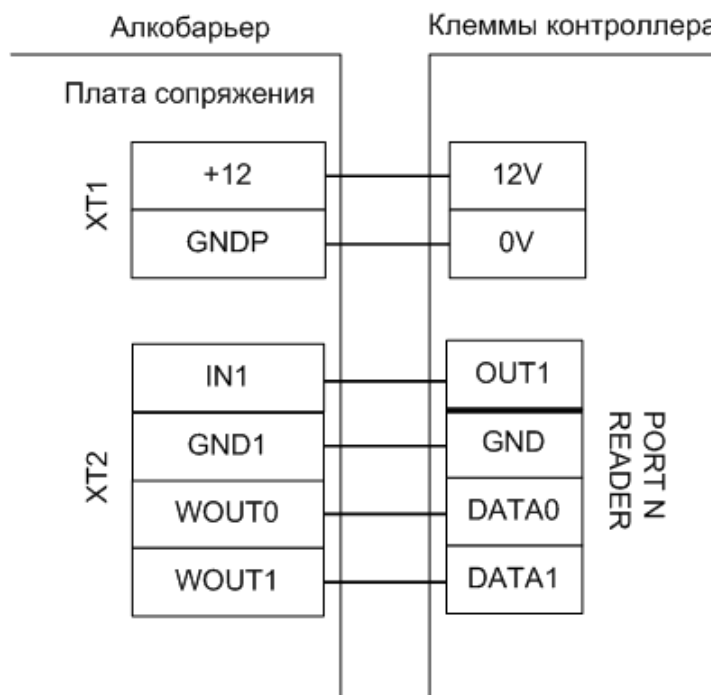
Схема подключения Алкобарьера.
