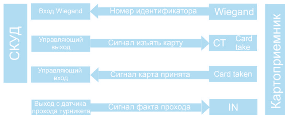
Рисунок 6.2.1 Алгоритм работы картоприемника
